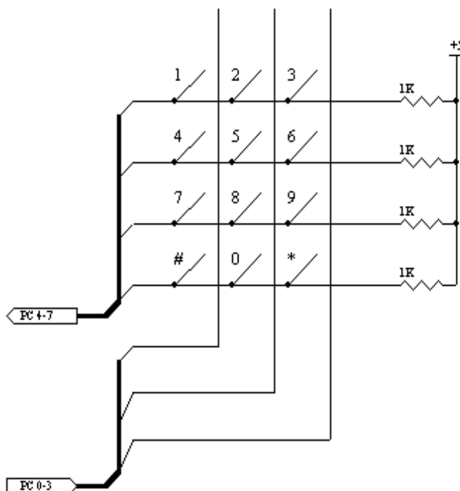
Gambar 2.1 Rangkaian Keypad
