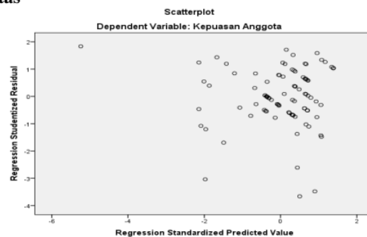
Gambar 2. Heteroskedastisitas
