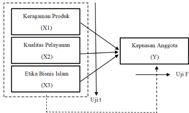
Gambar 1. Kerangka Penelitian
